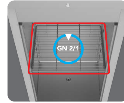
Daha Az Derinlik ile Daha Geniş GN 2/1 Raf Yerleşim Sistemi GN 2/1 Shelf Layout System with Less Depth and More Width
