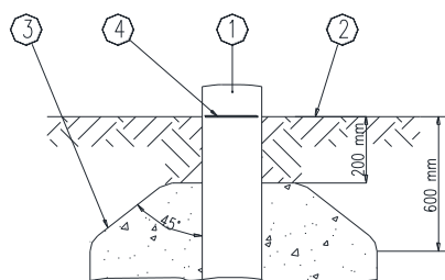
Fig. 2 – Detaliu fundație
