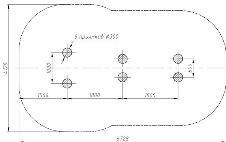
Fig. 3 – Plan de amplasare fundație
