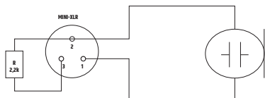
Condensateur sans résistance d'excursion interne.
