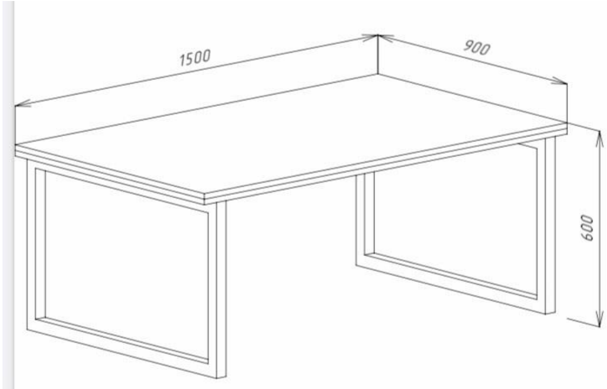
Masă pentru cantină
