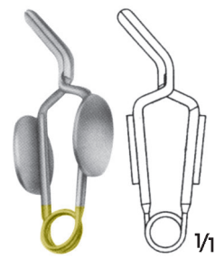
MÜLLER BG-1205 Kapama kuvveti 50 gr/Diz bükümlü Closing Forceps 50 gr/Knee-bent BG-1210 Kapama kuvveti 80 gr/Diz bükümlü Closing Forceps 80 gr/Knee-bent
