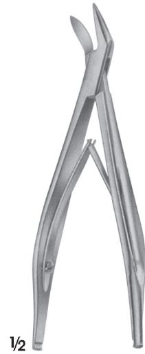
MICHEL BF-7422 Klip Uygulayıcı ve Çıkarıcı pens Clip applying and removing forceps 13 cm
