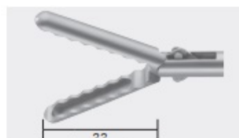
Fasszange, gewellt, Löffelform, doppelbeweglich, Ø 5 mm Grasping forceps, rippled, spoon shape, double action, Ø 5 mm
