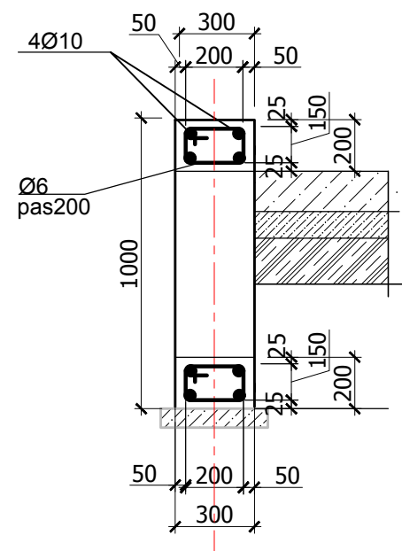
Secțiune fundație pavilion
