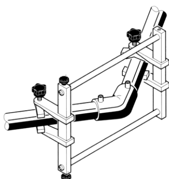
Fig. 2.3 COT LA 45° MONOFILAR BIFILAR
