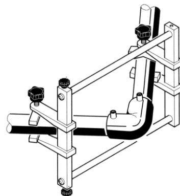
Fig. 2.2 COT LA 90° MONOFILAR
