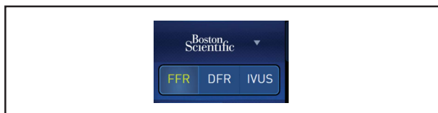
Figura 18. Selectați Modul
