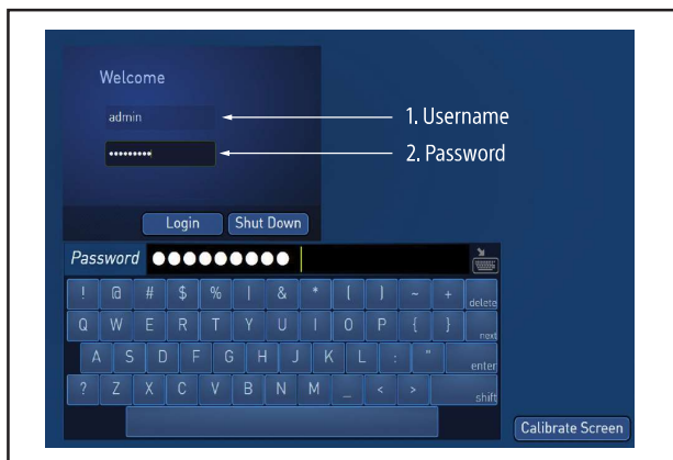
Figura 17. Autentificare
