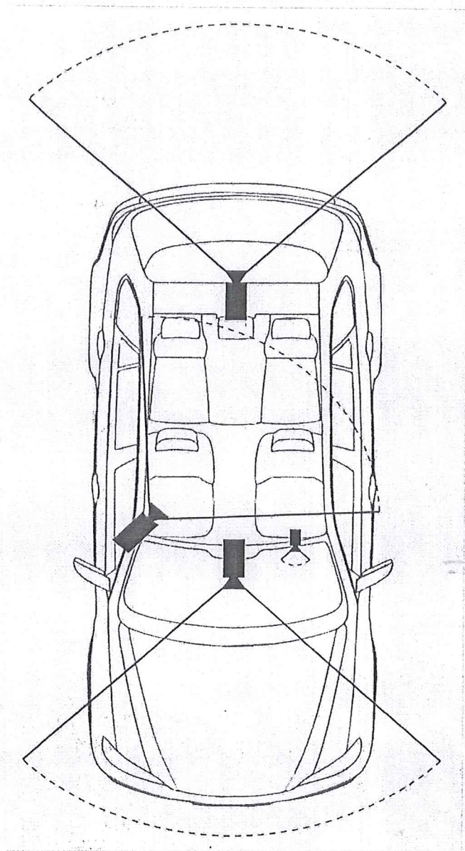
Schema amplasării camerelor video în autovehiculele speciale de examinare
