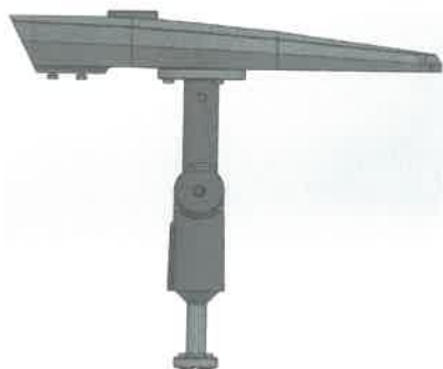
Fig. 3 – Modelul 3D al corpului de iluminat în poziția de încercare longitudinal orizontal ( \alpha_{xz} = 0^\circ și \beta_{xy} = 0^\circ )
