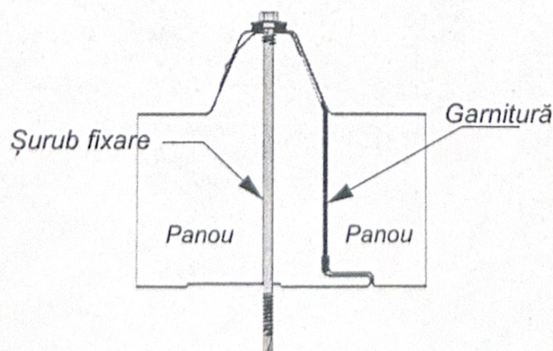
Secțiune panou acoperiș
