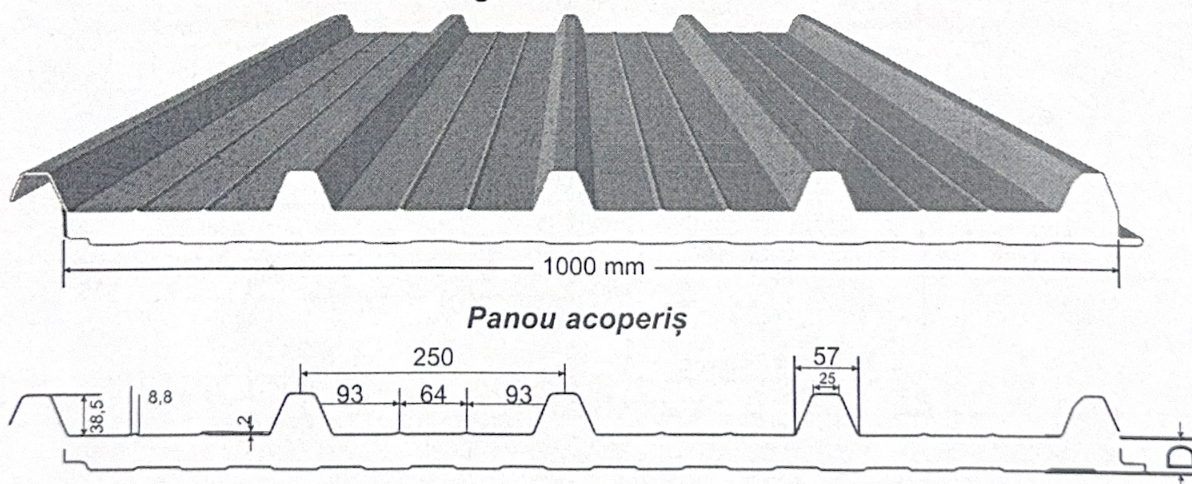
Secțiune panou acoperiș
