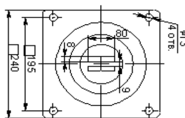
Чертеж № 4-Габаритные размеры изоляторов типа ИПУ-10/1600-12,5 УХЛ1
