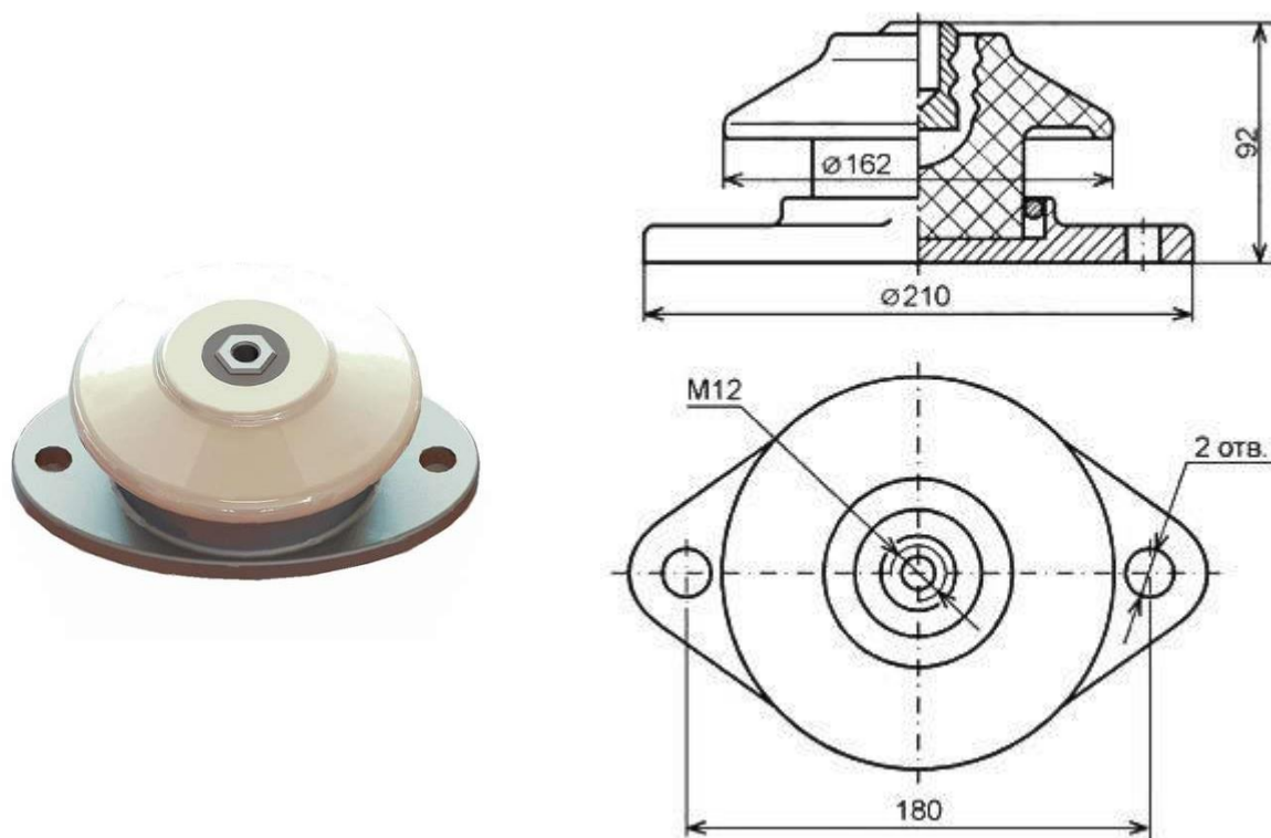
Чертеж № 6-Габаритные размеры изоляторов типа ИО-3-600-У1
