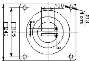
Чертеж № 5-Габаритные размеры изоляторов типа ИПУ-10/2000-12,5 УХЛ1
