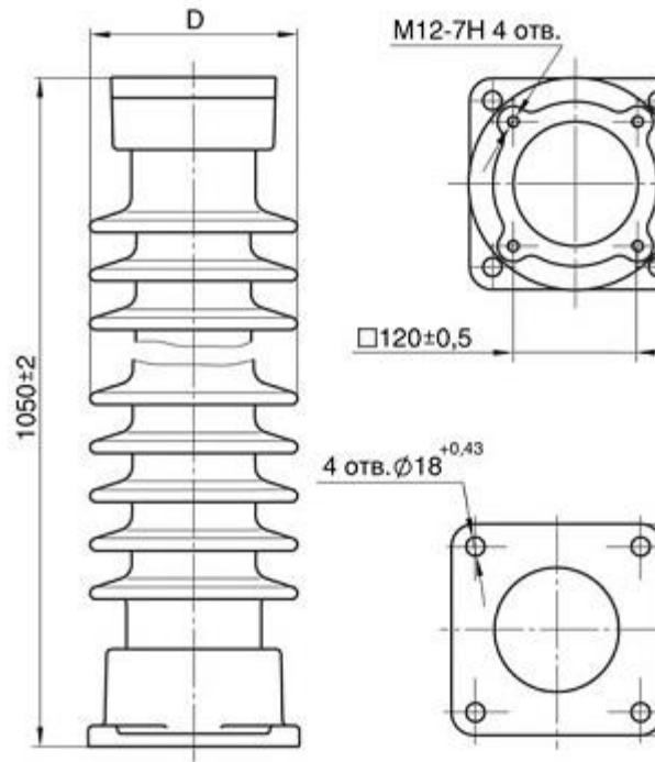
Чертеж № 9-Габаритные размеры изоляторов типа ИОС-110-400 I M УХЛ1
