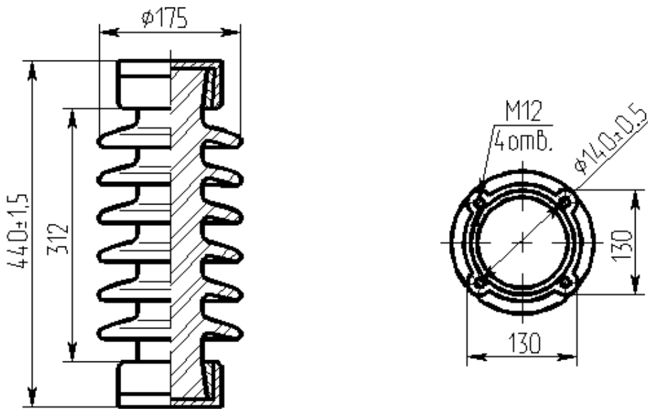
Чертеж № 8-Габаритные размеры изоляторов типа ИОС-35-500-01 УХЛ1
