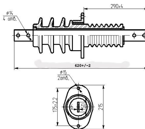
Чертеж № 1-Габаритные размеры изоляторов типа ИПУ-10 630-7,5 УХЛ1
