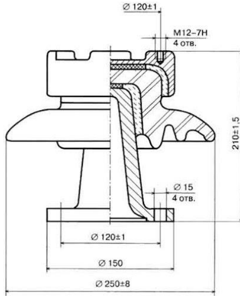
Чертеж № 7-Габаритные размеры изоляторов типа ОШН-20-80 УХЛ1
