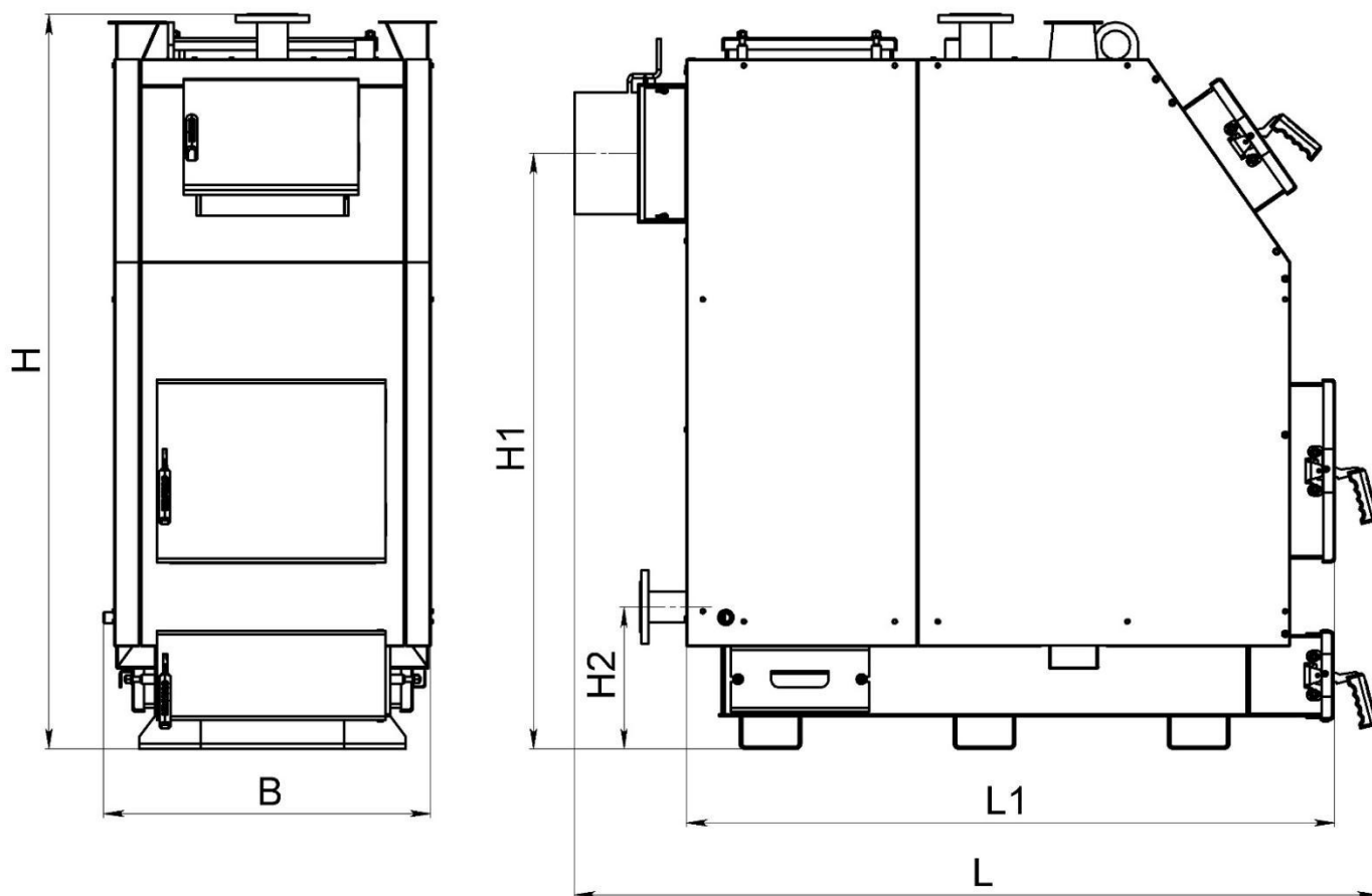
Рисунок 3.1 – Позначення габаритів
