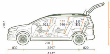
PROFIL 7 LOCURI
