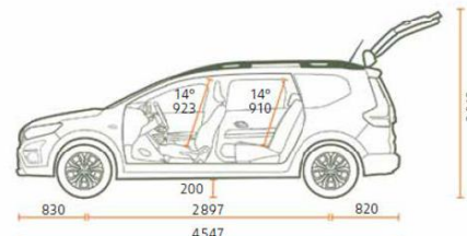
PROFIL 5 LOCURI
