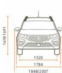
VEDERE FRONTALĂ
