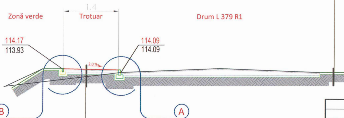
Secțiune 5 - 5
