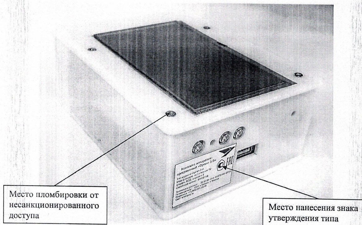
Рисунок 5 – Блок обработки данных комплексов аппаратно-программных «Орлан 3.0» (исполнение 02, вариант 2)
