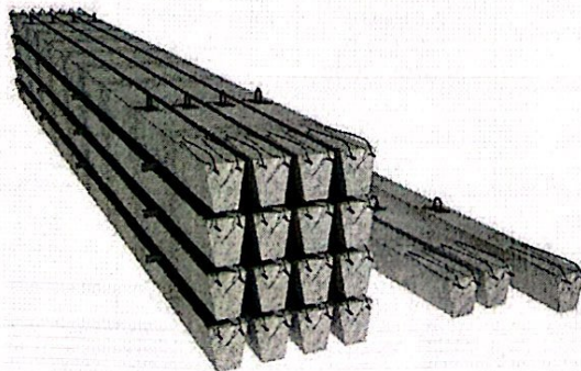
Exemplu schița comună Stâlp SET 10,5; SET 9,5; SET 7,5
