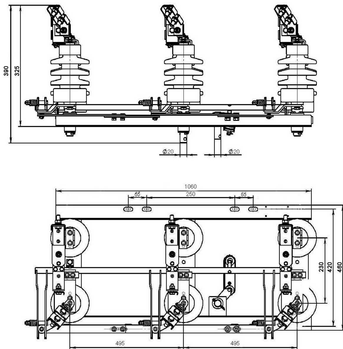
Рисунок 12.5.1. Линейный разъединитель наружной установки РЛНДЗ-10/400 У1
