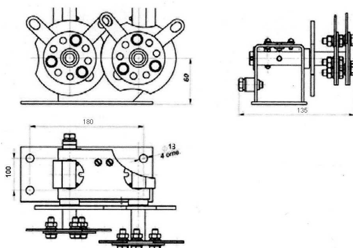
Рисунок 12.5.2. Привод ПРЗ-10 У1
