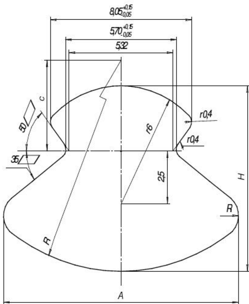
Рисунок 2 - Размеры фасонного овального провода
