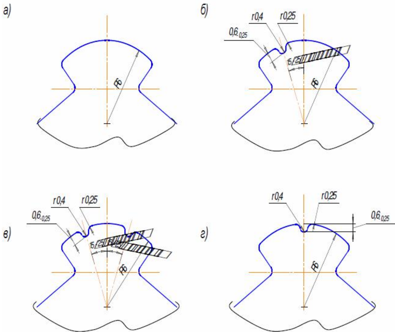
Рисунок 3 - Отличительные признаки поперечного сечения провода
