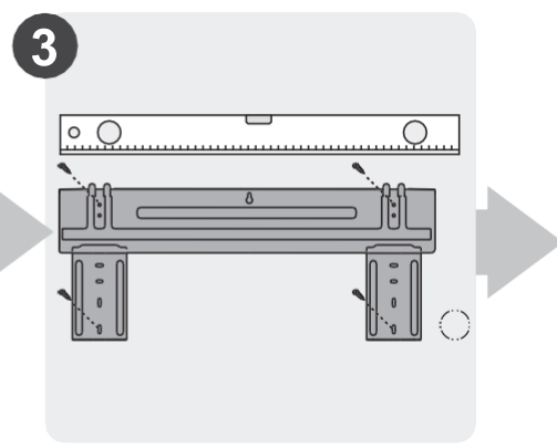
3 Atașați placa de fixare
