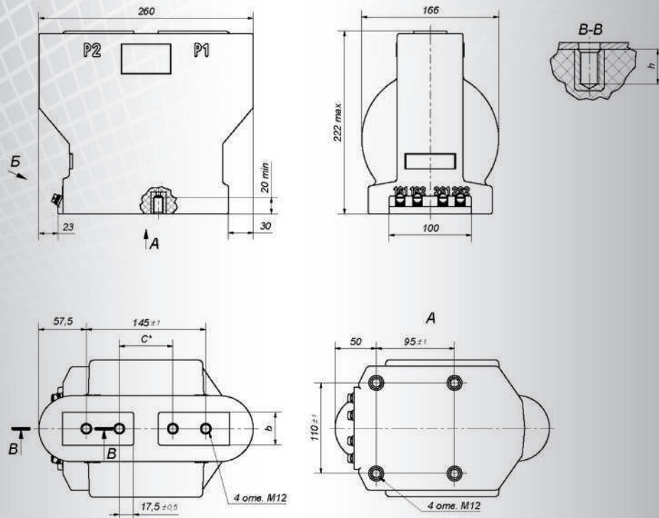
Рисунок 1 – Габаритне креслення трансформатора струму ТОЛУ-10
