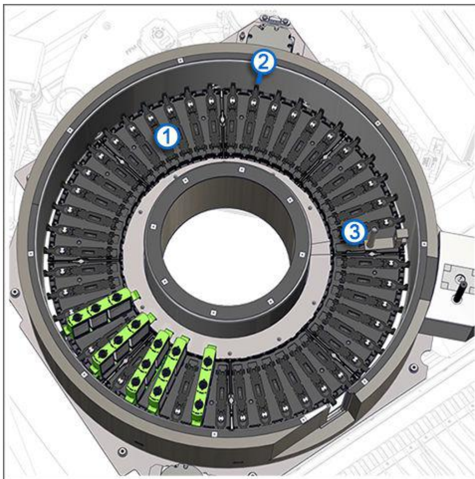
Figură 81: Carusel de reactivi (Alinity i)
