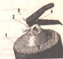
Рис.1 1. Основной корпус, 2. Индикатор давления, 3. Запорно-пусковое устройство (ЗПУ), 4. Чека, 5. Насадка (рукав)
