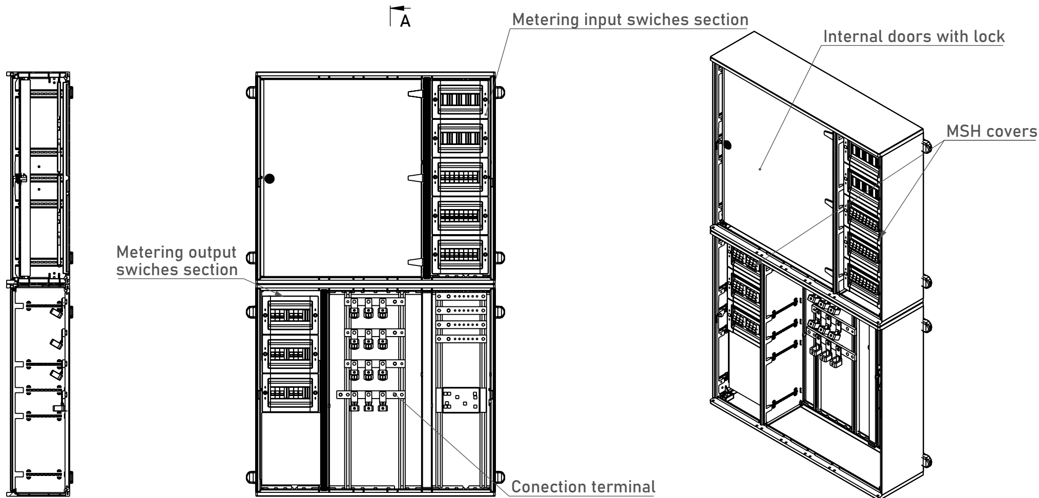
SECTION A-A
