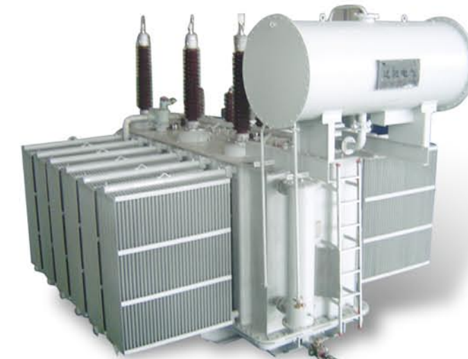
110kV牵引变压器 110kV Traction Transformer
