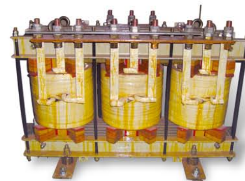
船用变压器 Marine Transformer
