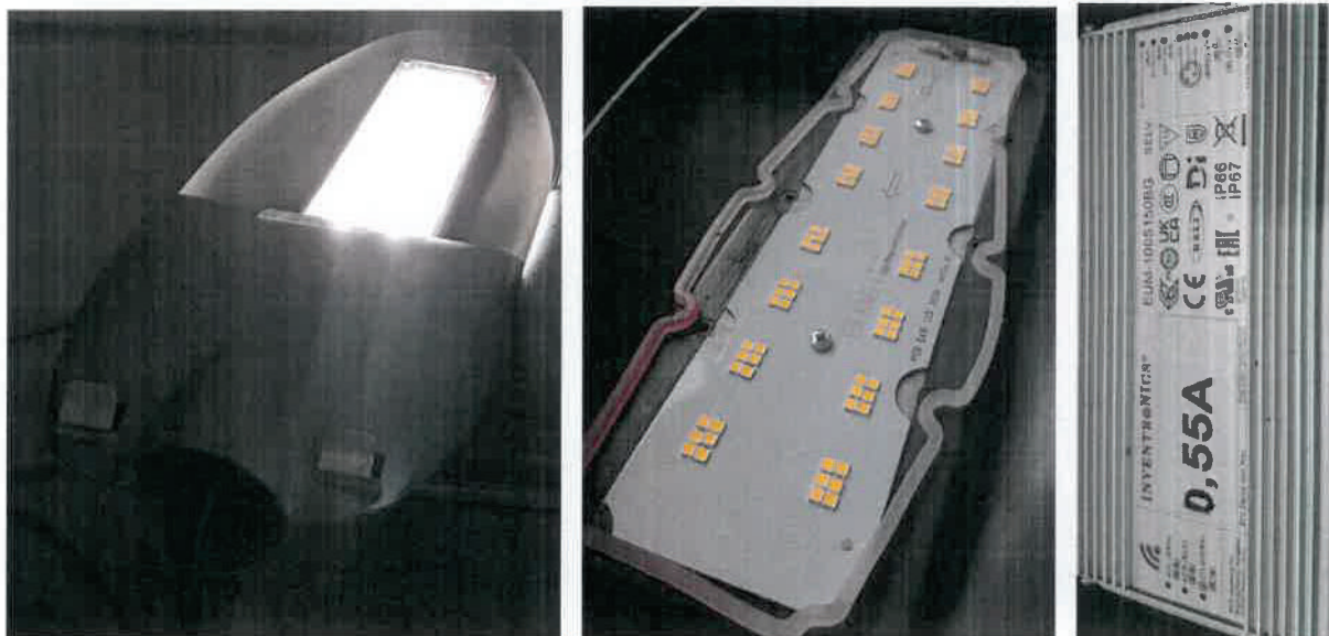
Fig.2 Poze produs CIL după test
