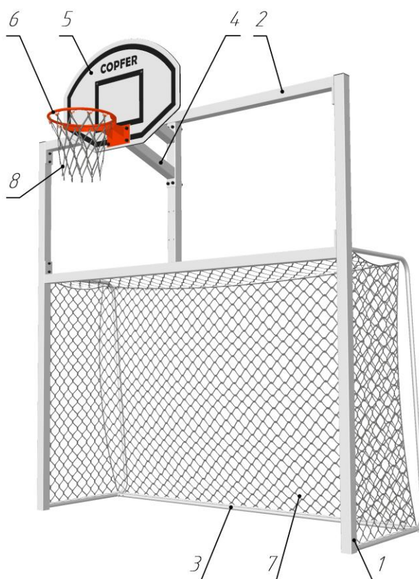
Рис.1 Общий вид ворот комбинированных РТР 712
