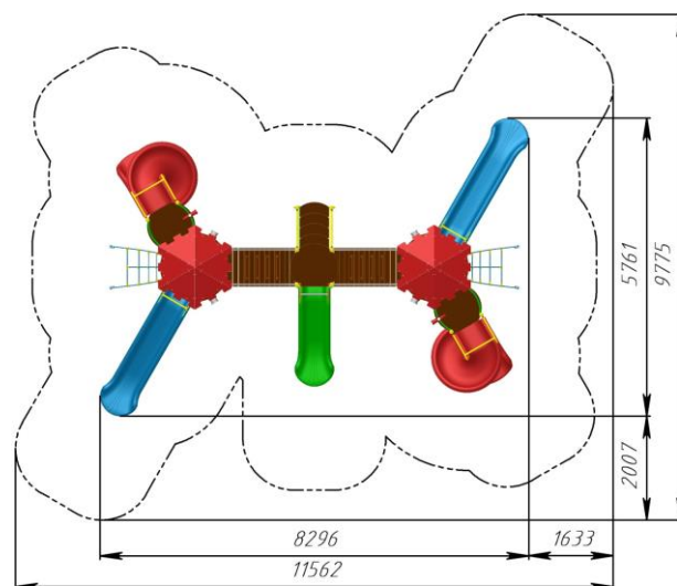
Fig. 1 – Spațiu minim de siguranță
