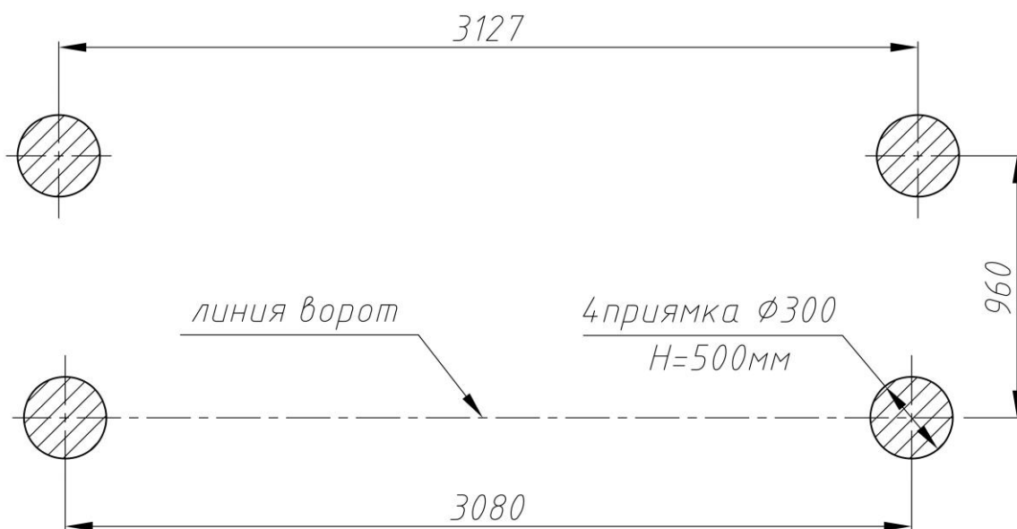
Рис.2 План фундамента ворот комбинированных РТР 712
