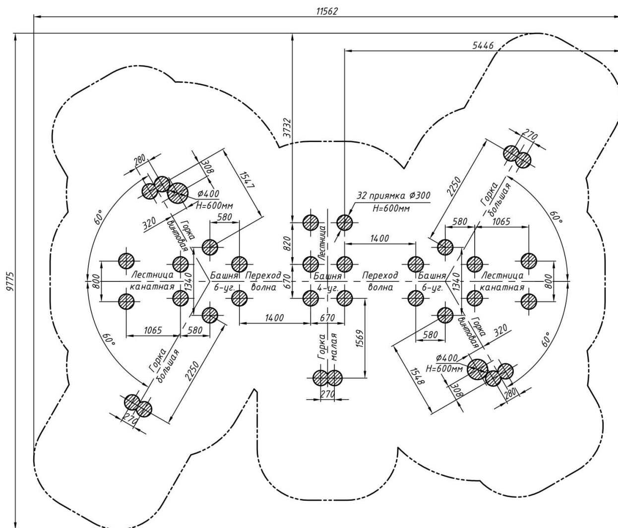
Fig. 2 – Plan de amplasare fundație
