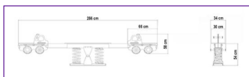
Vedere laterala:
