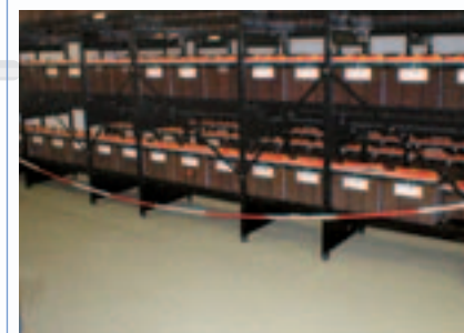
Рис. 23 Смонтированные батареи Classic Energy Bloc
