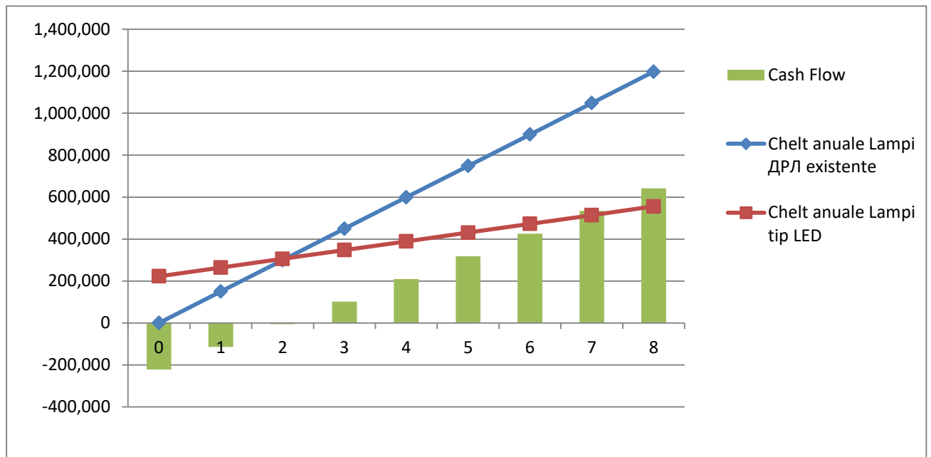
Figura 12 Rezultatul economico financiar al măsurii 2 Existent vs LED
