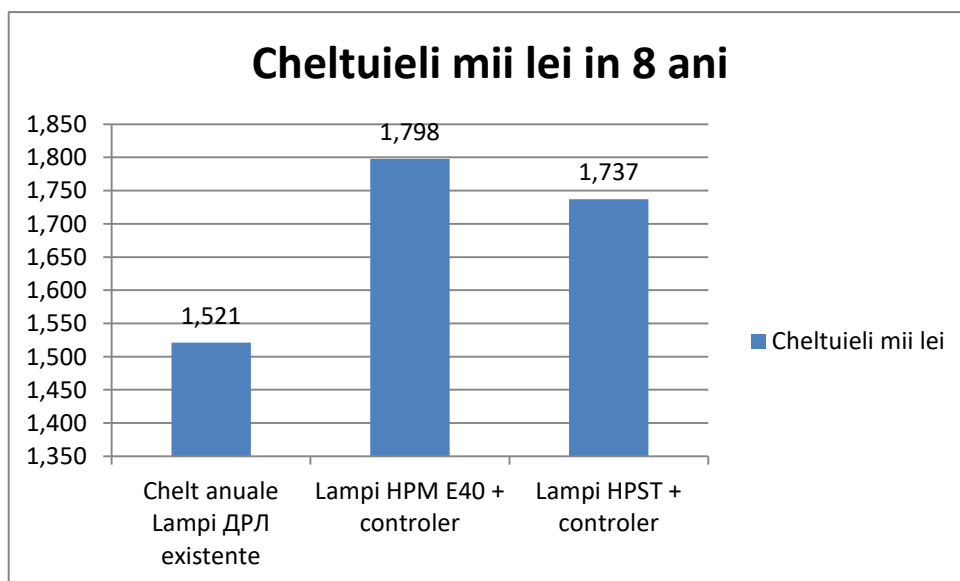
Figura 18 Cheltuielile cumulate al măsurilor combinate pentru anul 8 în mii lei
