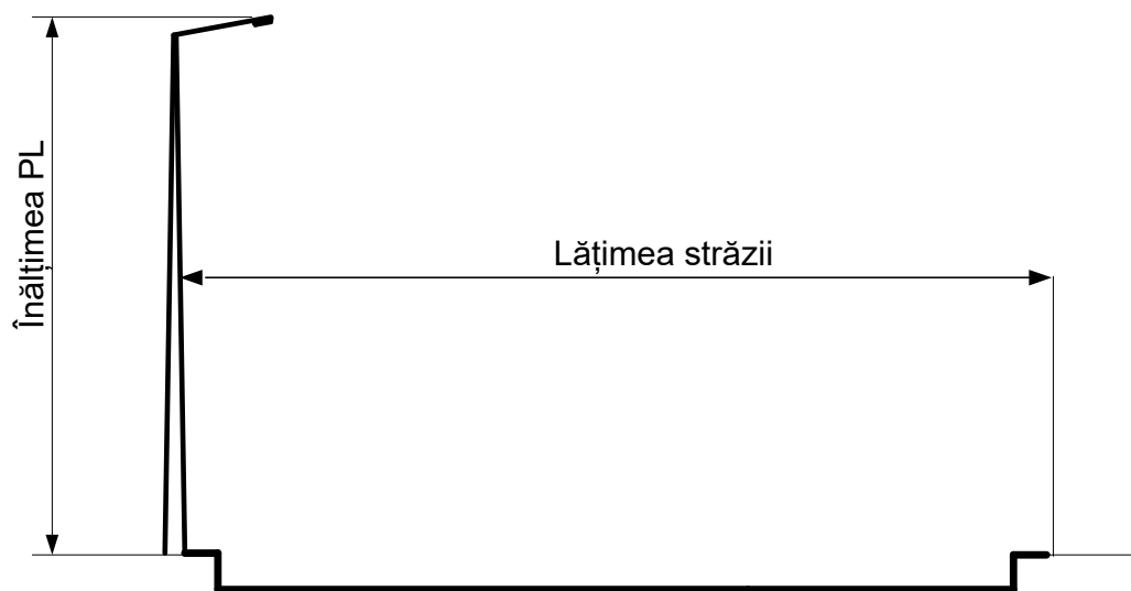
Figura 2 Schema amplasamentului sistemului de iluminat străzile localității cu mărimi calculate medii
