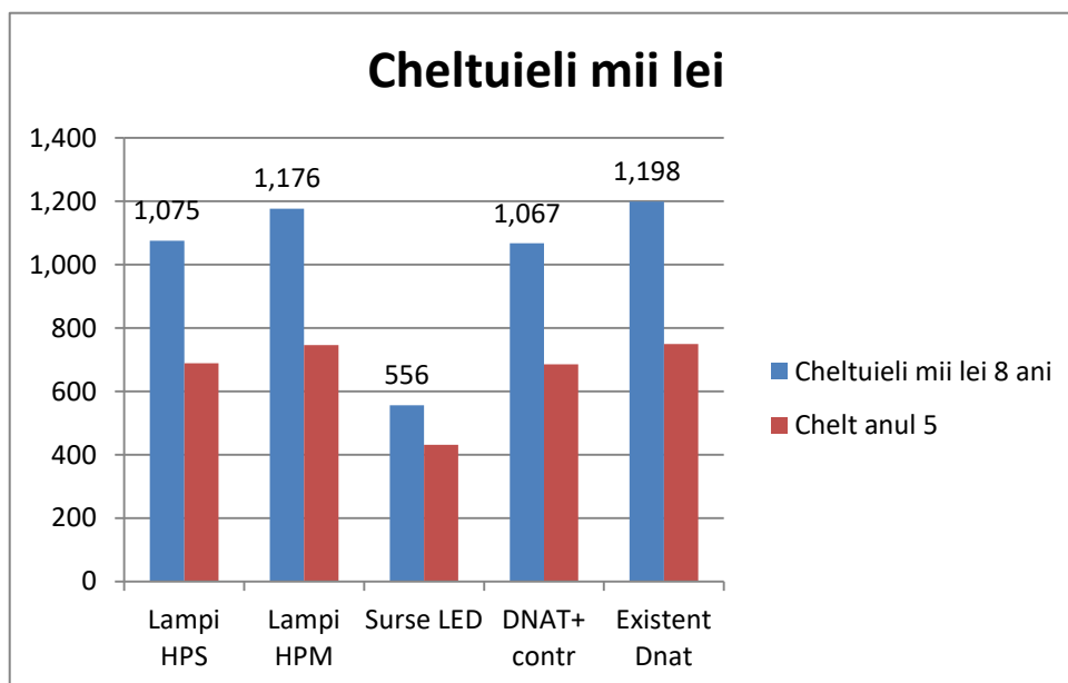
Figura 17 Cheltuielile cumulate al măsurilor 1-4 pentru anul 5 și anul 8 în mii lei
