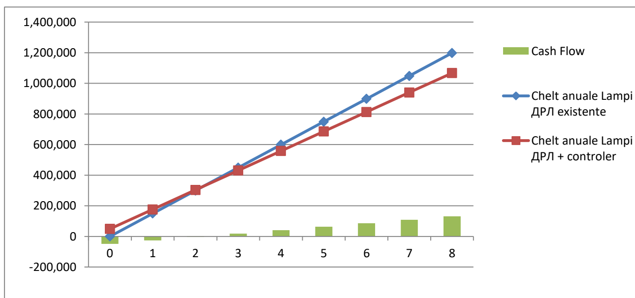
Figura 15 Rezultatul economico financiar al măsurii 4 Existent vs ДРЛ + controler
