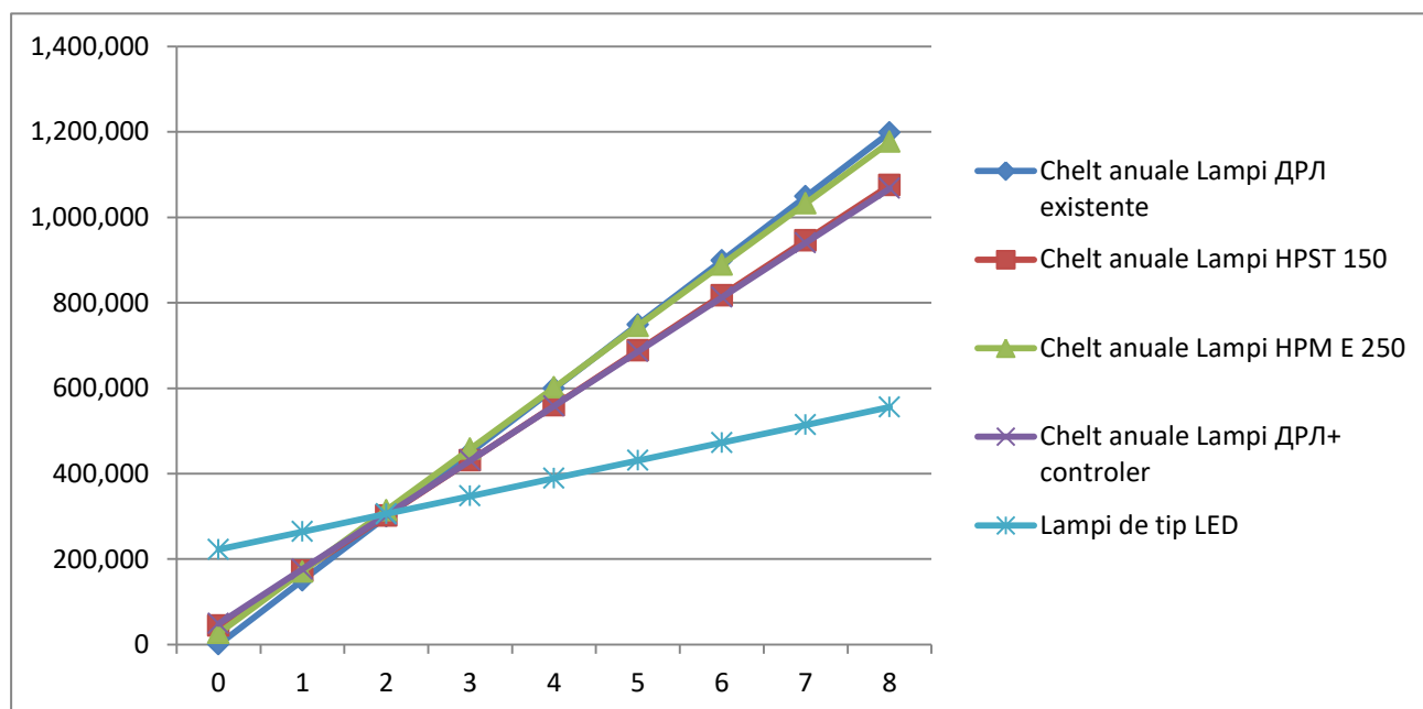
Figura 16 Rezultatul economico financiar al măsurilor 1-4
