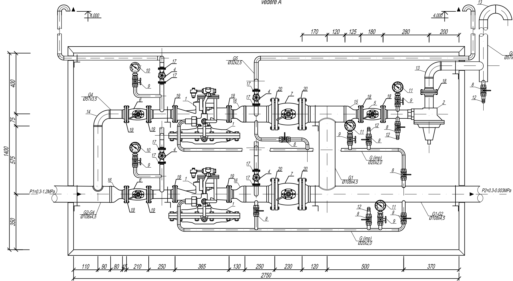
SCHEMA TEHNOLOGICA S 1:10 vedere A
