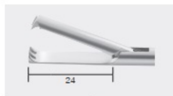
Krallengreifer, 2 x 3 Zähne, einfach beweglich, Ø 5 mm Claw grasping forceps, 2 x 3 teeth, single action, Ø 5 mm
