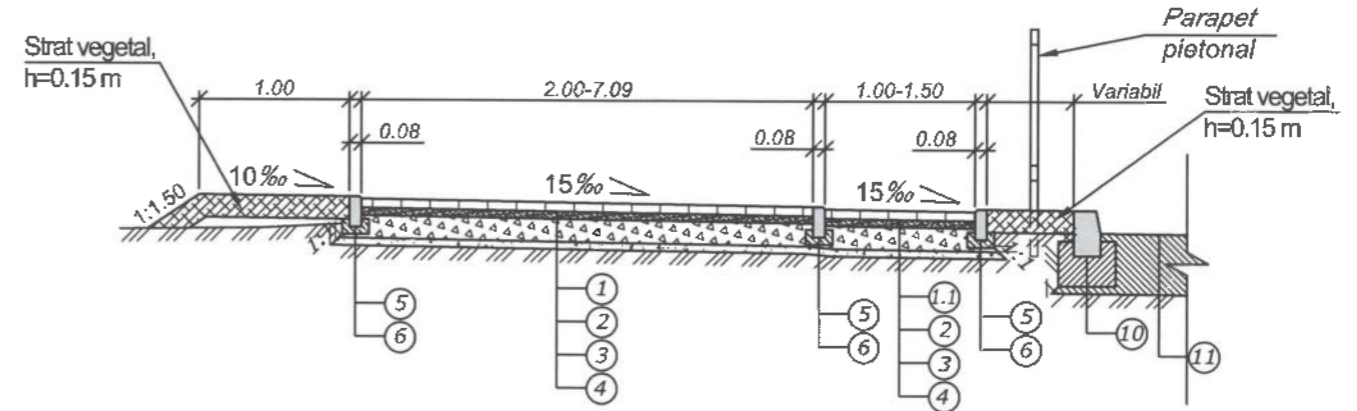
Profil transversal Tip IV de execuție a îmbrăcămintei rutiere
