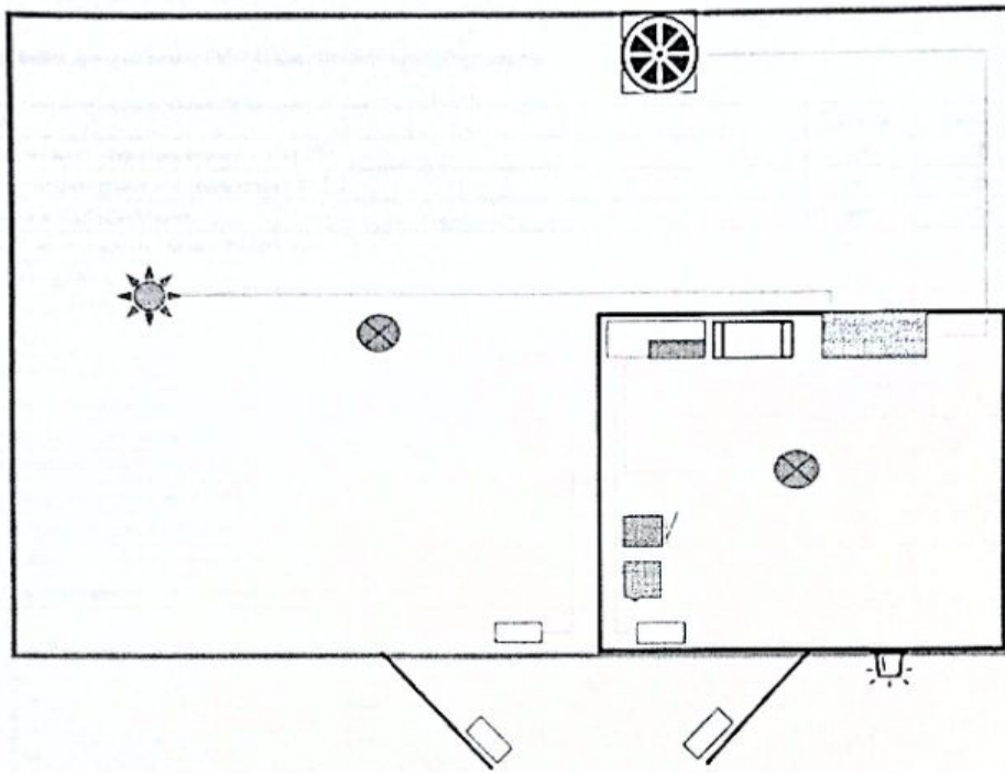
Схема блок- бокса хроматографа
