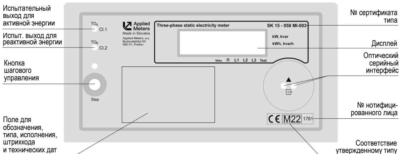
Пример лазерной печати на крышке
