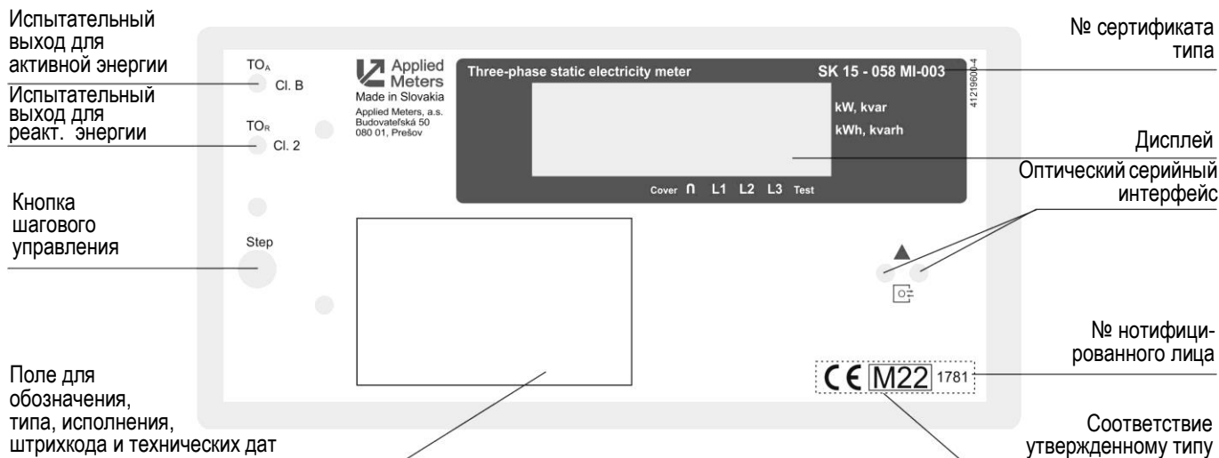
Пример щитка счётчика в корпусах E и 9
