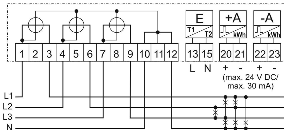
АМТ В2х-FA4Т9IE с внешним управлением тарифов, с импульсными выходами энергии +А и –А
