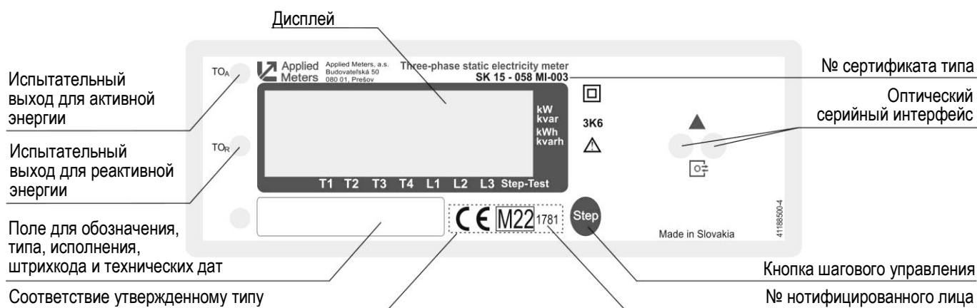
Пример щитка счётчика в корпусе С
