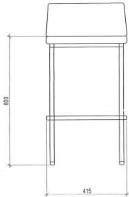
VEDERE FRONTALA , Sc. 1:10
