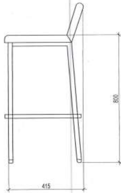
VEDERE LATERALA , Sc. 1:10
