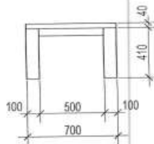
VEDERE LATERALA , Sc. 1:50
