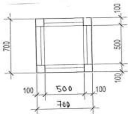
PLAN MASA DE CAFEA , Sc. 1:50
