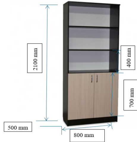
FIG 2 „Dulap pentru dosare cu rafturi”
