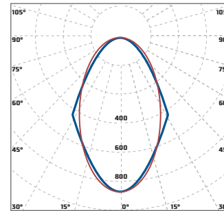
«Diora Unit К60» глубокая КСС 60°
