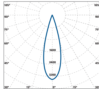
«Diora Unit К30» концентрированная КСС 30°
