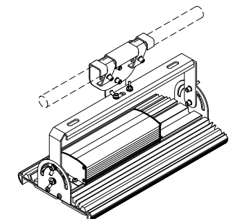
Тросовый подвес (до Ø20 мм)
