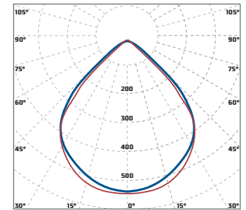
«Diora Unit Г90» глубокая КСС 90°
