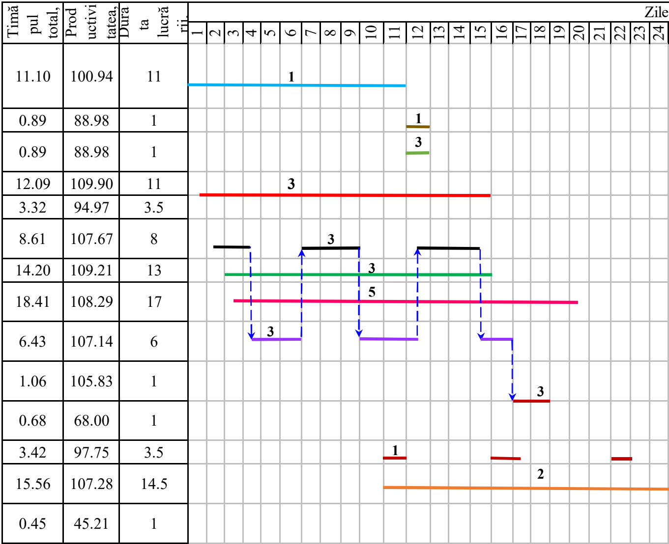
graficul calendaristic de execuție a lucrărilor de montare a rețelei exterioare de canalizare
