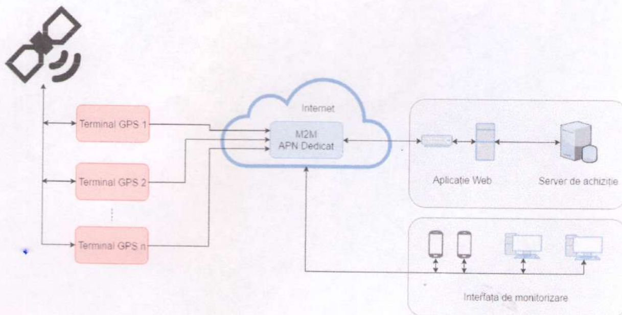
Figura 1 Schema funcțională a sistemului de monitorizare.
