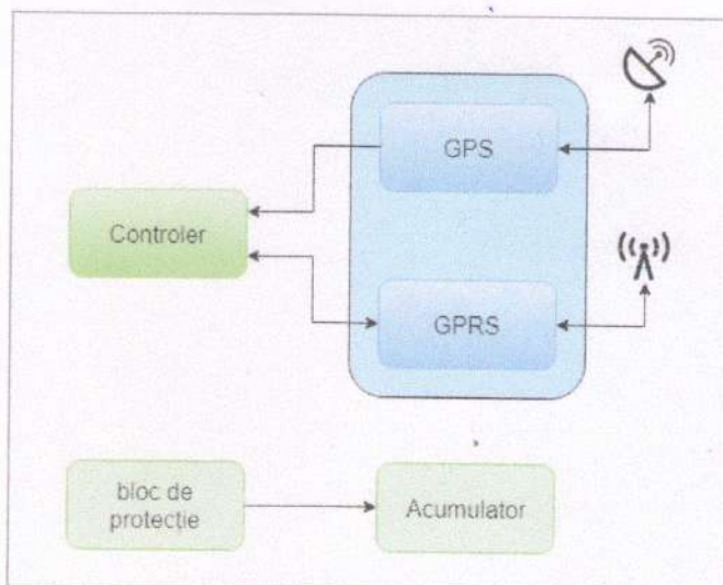
Figura 2 Schema bloc a terminalului mobil GPS.
