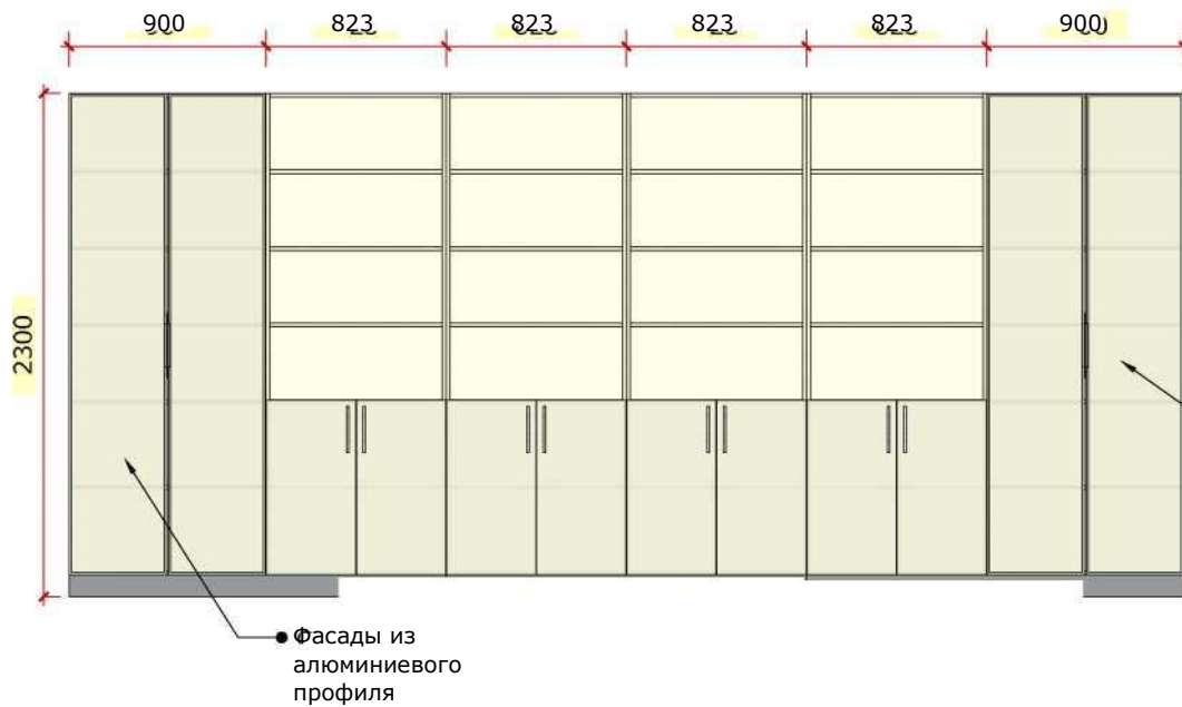
Вид спереди
