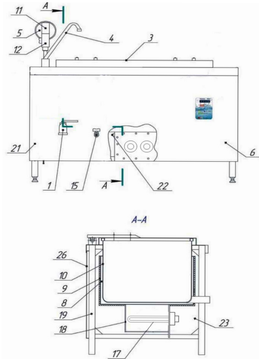
Рис. 1. Загальний вигляд котла
