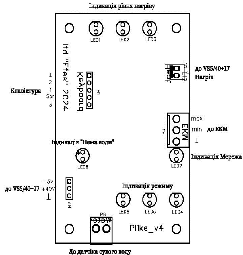
Додаток М Схема електрична з'єднань плати керування PL1ke
