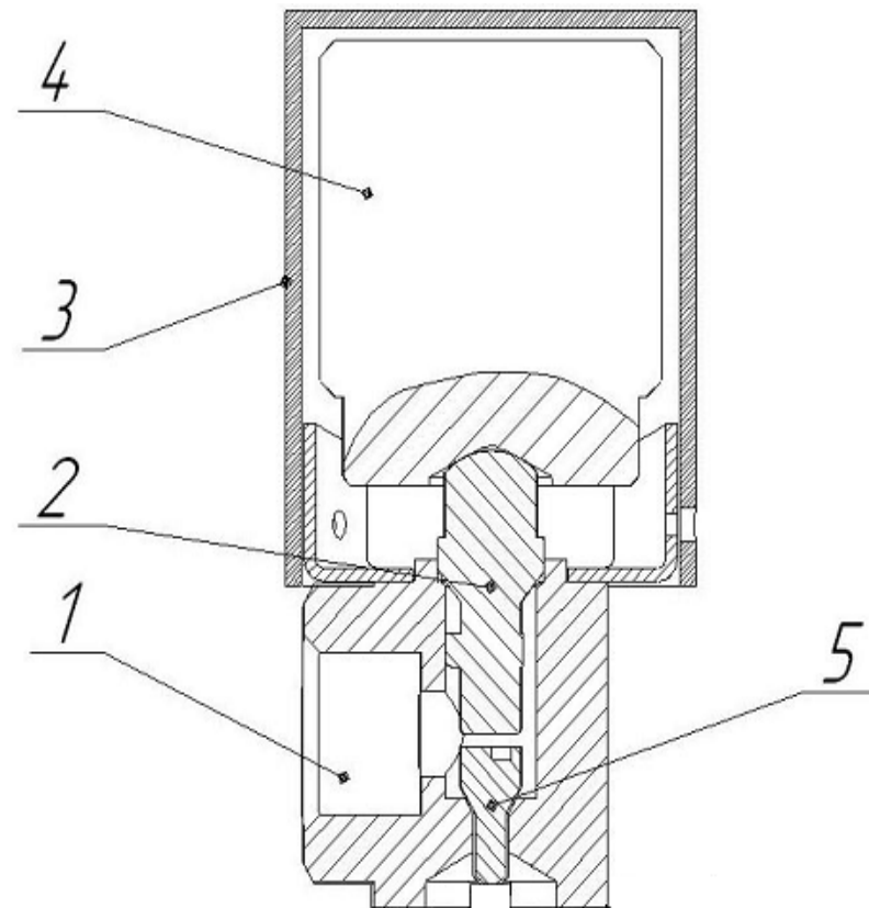
Рис. 2. Запобіжний клапан
