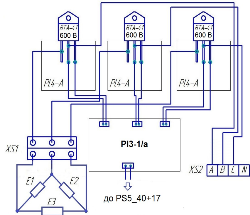
Додаток Г Принципова електрична схема підключення плати PL3-1/a і силових плат PL4-A котла моделі KE-60
