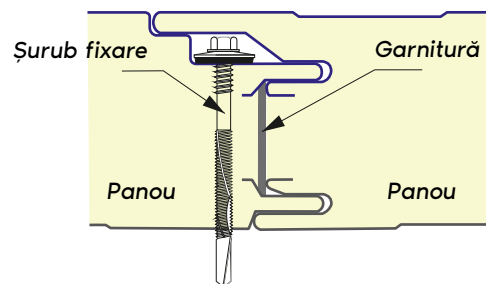
Secțiune prindere panouri
