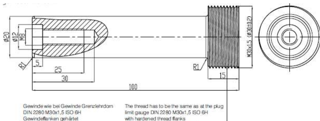
Fig. 10 – Test object
